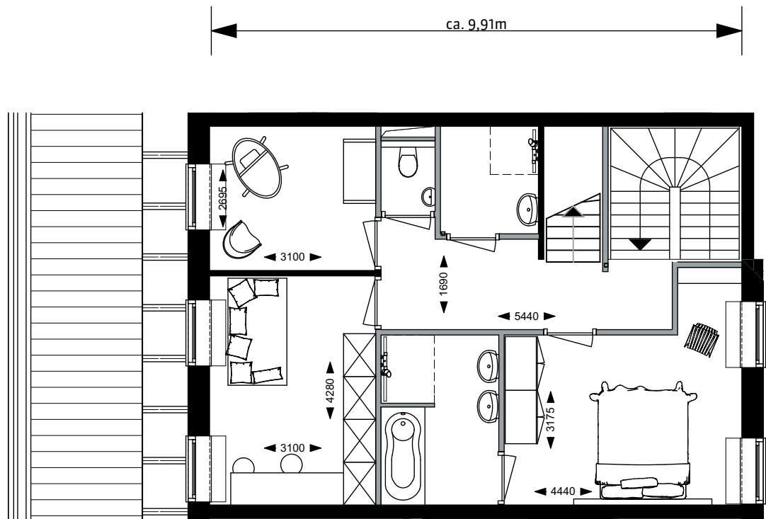
F.09 1e verdieping
