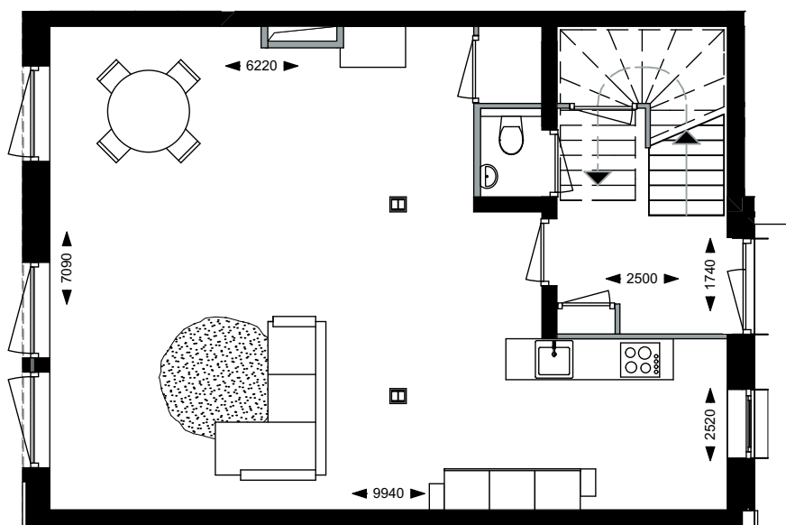
F.09 begane grond
