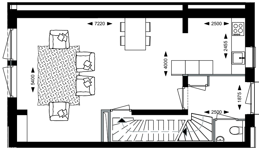
F.07 begane grond
