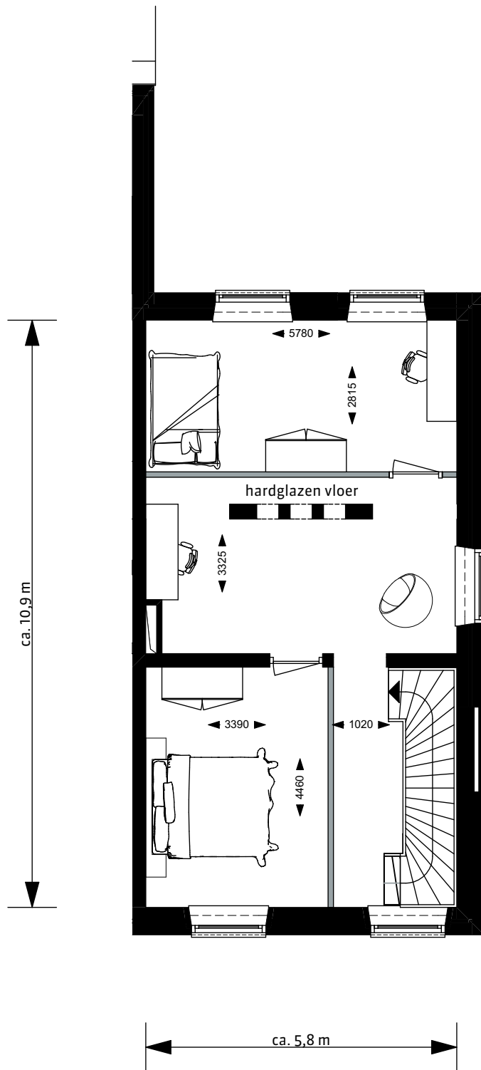
Trappenhuis 1e verdieping
